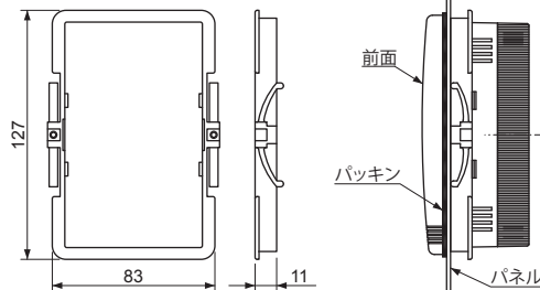
パネル取付パーツ (パッキン付)
