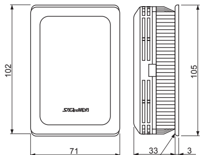
湿度センサ (HEK-I1R001)
