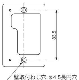
センサ取付板
